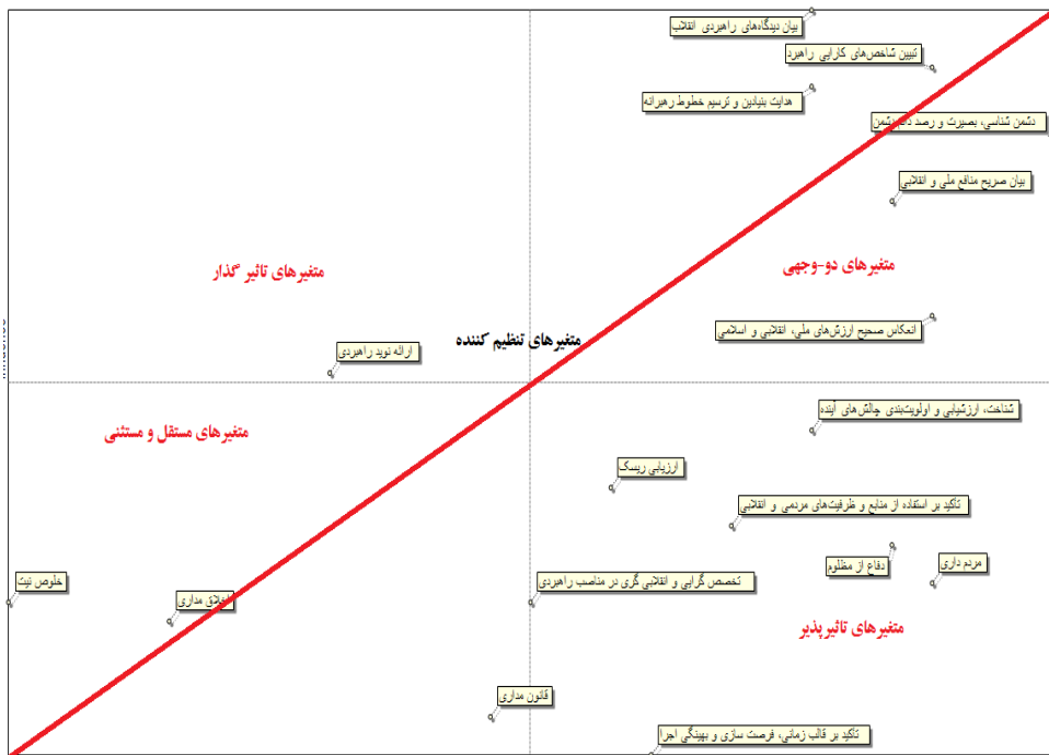
شکل شماره (۲): ماتریس تأثیرات مستقیم و متغیرهای کلیدی (خروجی نرم افزار میک‌مک)
