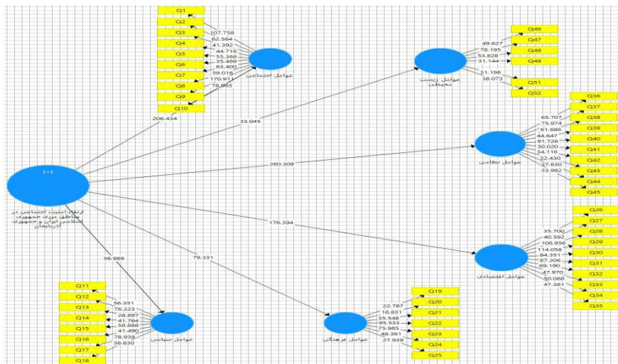
شکل ۳: مدل اندازه‌گیری انعکاسی اصلاح‌شده در حالت معناداری ضرایب
