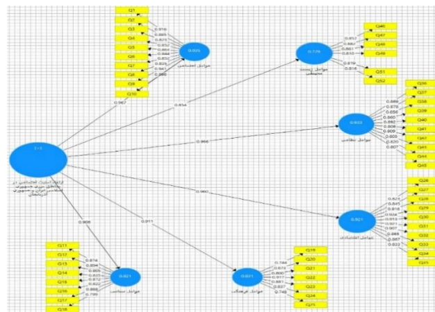
شکل ۲: مدل اندازه‌گیری انعکاسی اصلاح‌شده در حالت تخمین ضرایب
